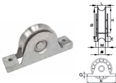
A318080 Roue à support à encastrer gorge ronde
