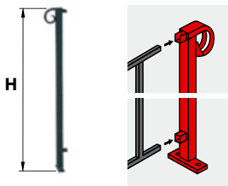
Poteau balcon départ à visser
