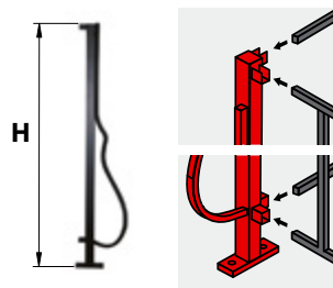
Poteau balcon à angle lombarde à visser
