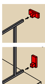
Platine à visser pour poteau balcon (x2)
