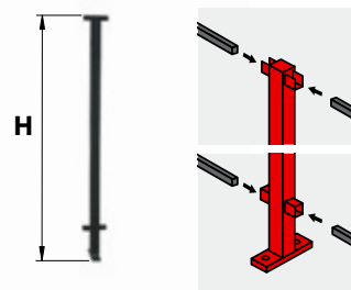
Poteau balcon jonction à visser
