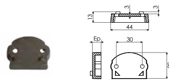
J0535.. Rehausse de gâche pour RY59
