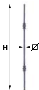
BAF135.. Barreau fantaisie double 135
