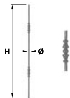
BAF150.. Barreau fantaisie double 150
