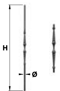
BAF141.. Barreau fantaisie 141
