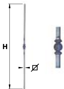
BAF153.. Barreau fantaisie 153
