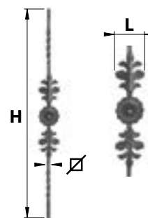
BAF78.. Barreau fantaisie 78
