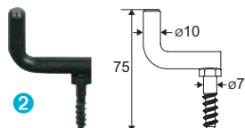
0720046 - Coudé à vis
