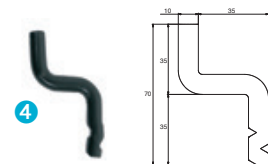
0720024 - Coudé à sceller
