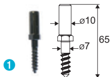
0720054 - Droit à vis
