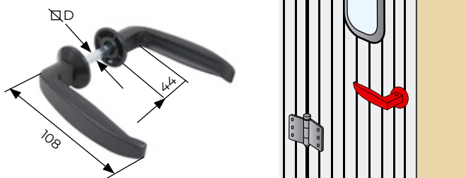
Béquille double saillie
