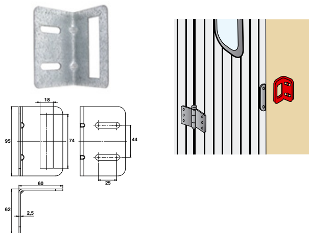
Gâche de serrure 2 lumières
