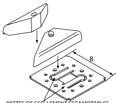
PATTES DE SCELLEMENT ESCAMOTABLES
