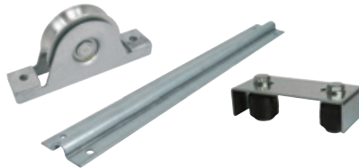
Ferrures pour portails coulissants acier, alu et PVC
